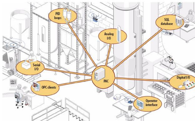
Fig. 4.3-2 (Fonte: OPTO 22)
